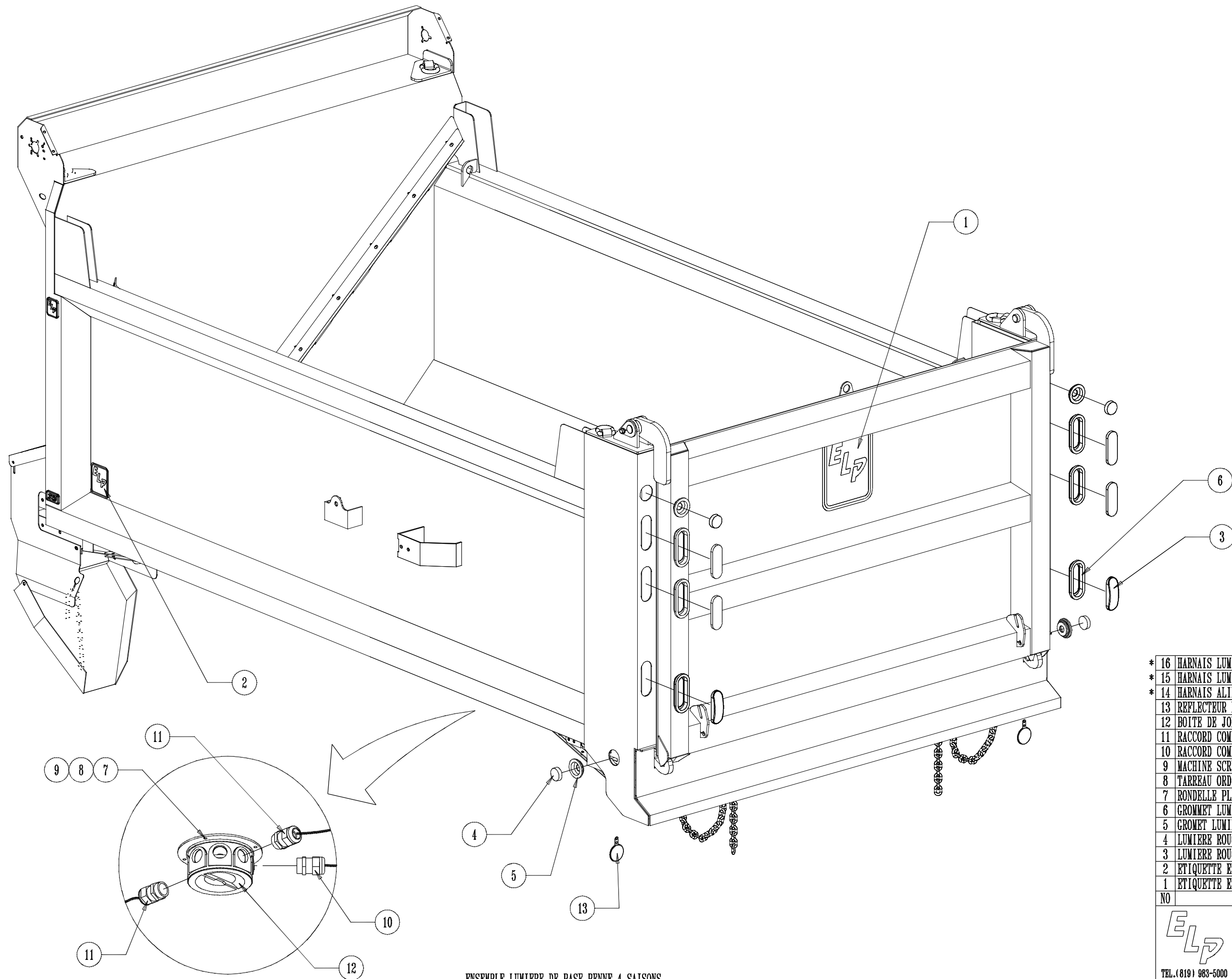
ENSEMBLE LUMIERE DE BASE BENNE 4 SAISONS
