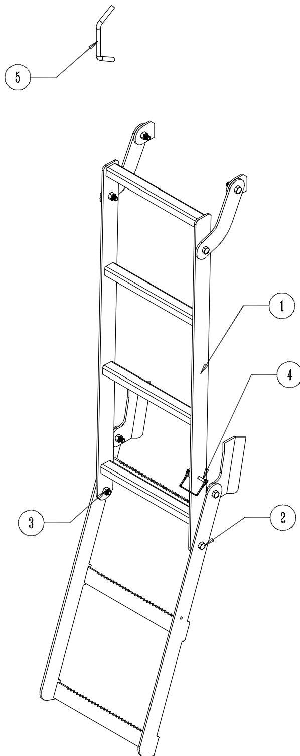
ENSEMBLE FINITION ECHELLE RETRACTABLE GAUCHE / LEFT FOLDABLE LADDER FINITION ASSEMBLY
