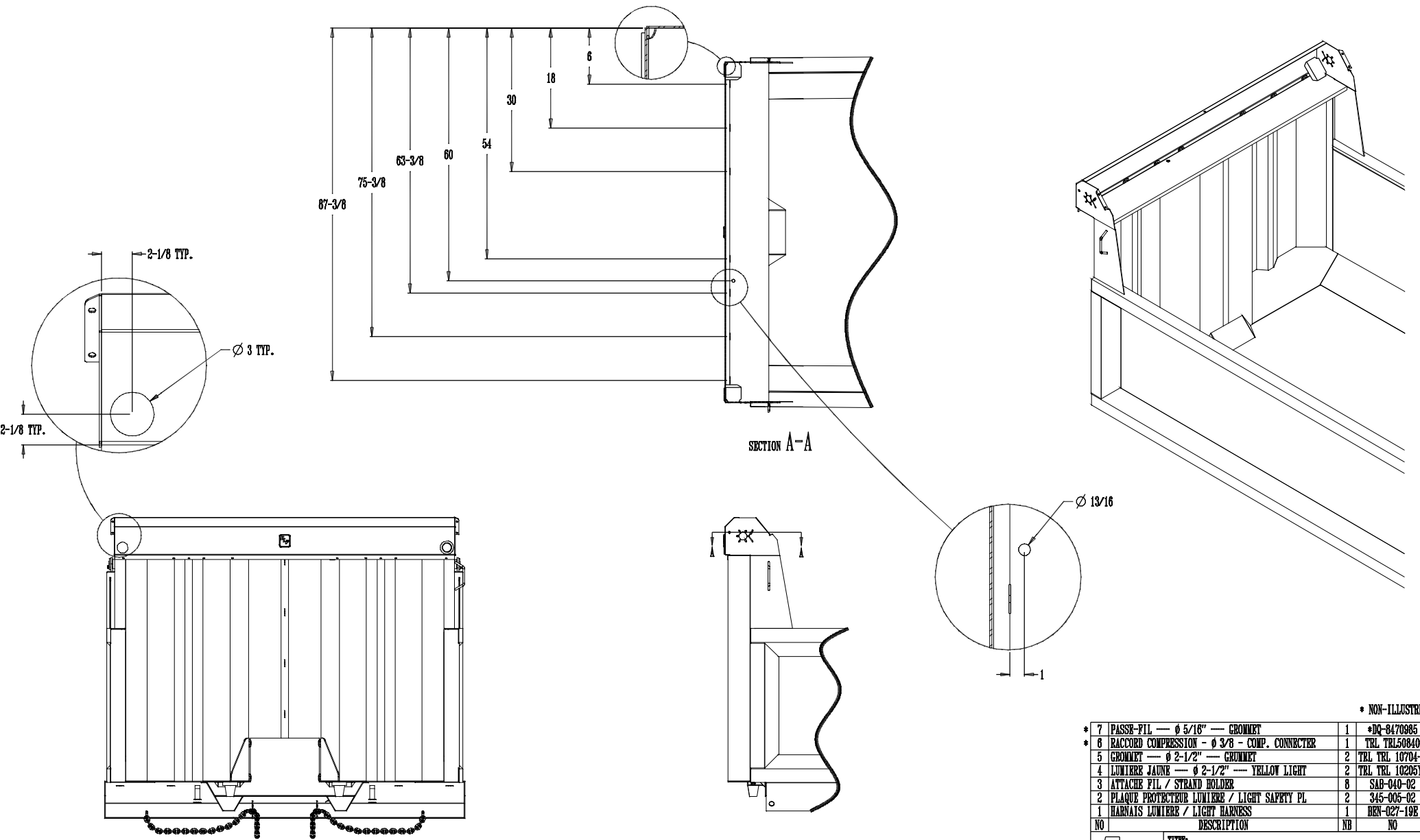
SOUDURE COMPLETE
