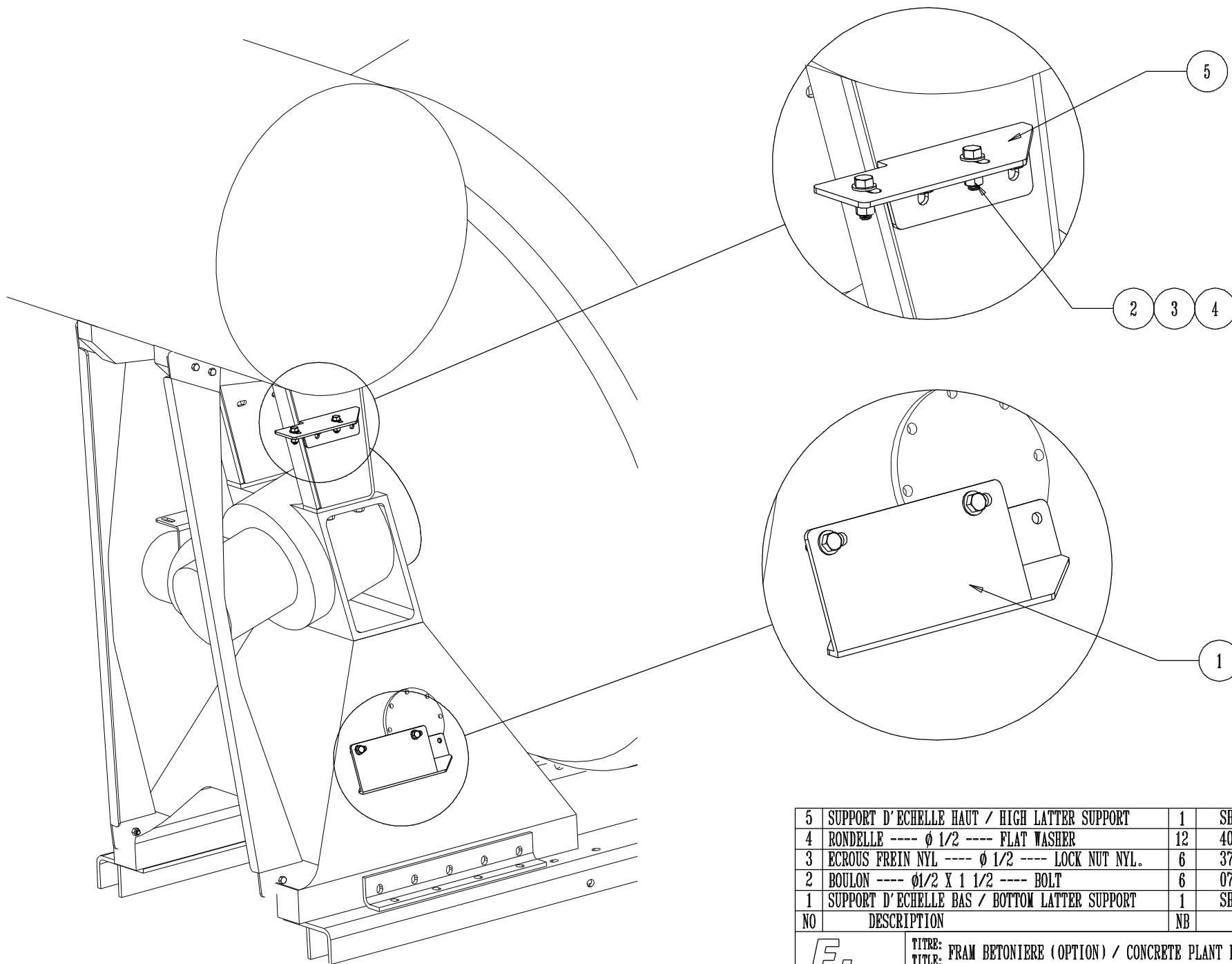
ENSEMBLE SUPPORT D'ECHELLE "LONDON" AVEC QUAINCAILLERIE / WITH HARD WARE "LONDON" LADDER SUPPORT ASSEMBLY
