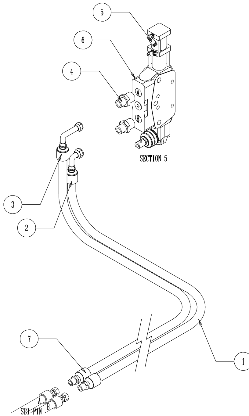
SECTION VALVE POUR PIN SBI/SBI PIN VALVE SECTION
