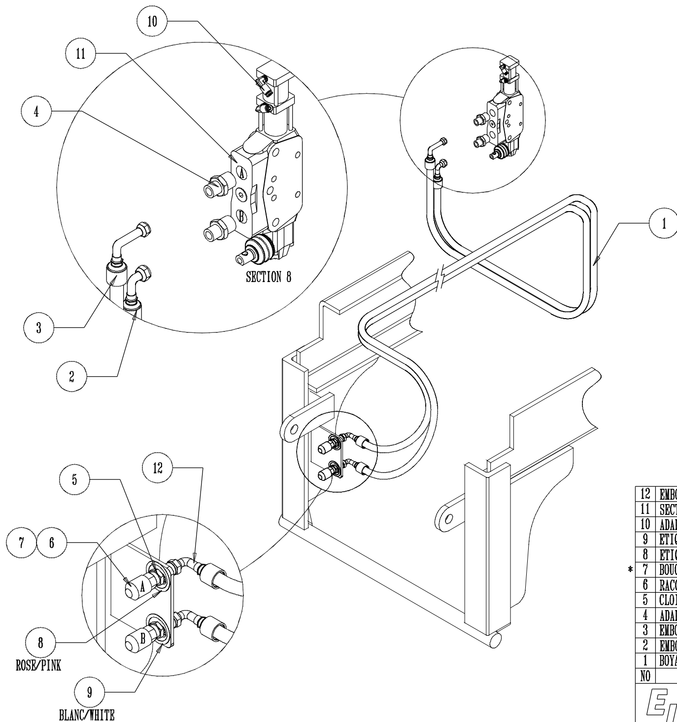
SECTION VALVE POUR LAME ARRIER GA-DR/R-L REAR BLADE VALVE SECTION
