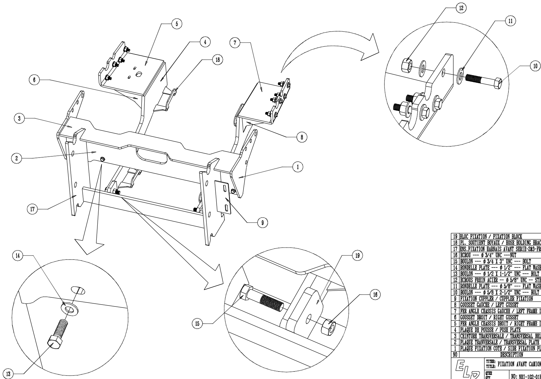
ENSEMBLE POUR MACK CTP ESSIEUX AVANCE / WHEEL SHAFT MACK CTP ASSEMBLY
