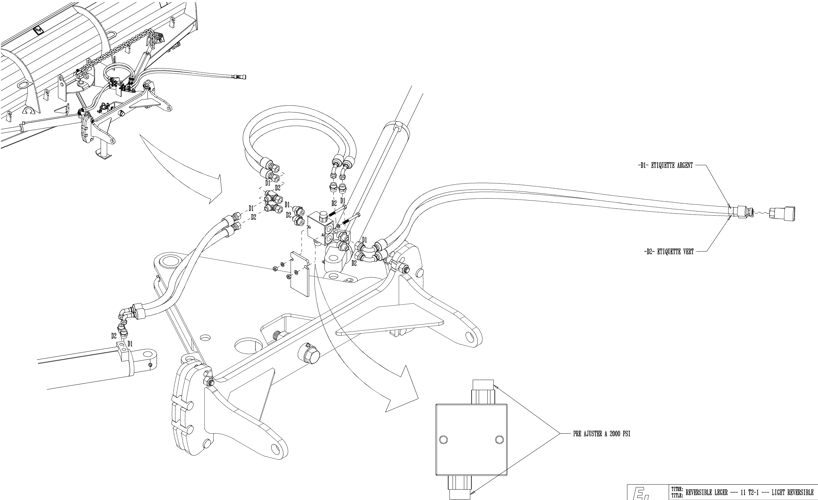
MONTAGE HYDRAULIQUE
