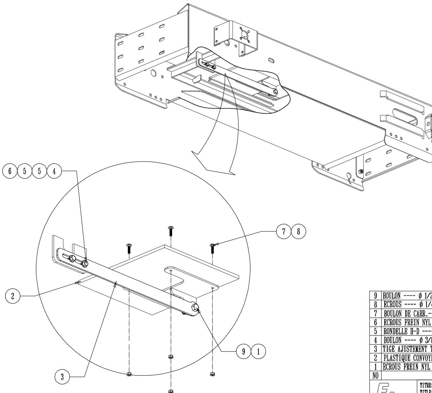
ENSEMBLE FINITION CONVOYEUR AVEC TRAPPE MECANIQUE / MECANIC TRAPPED CONVEYOR FINITION ASSEMBLY
