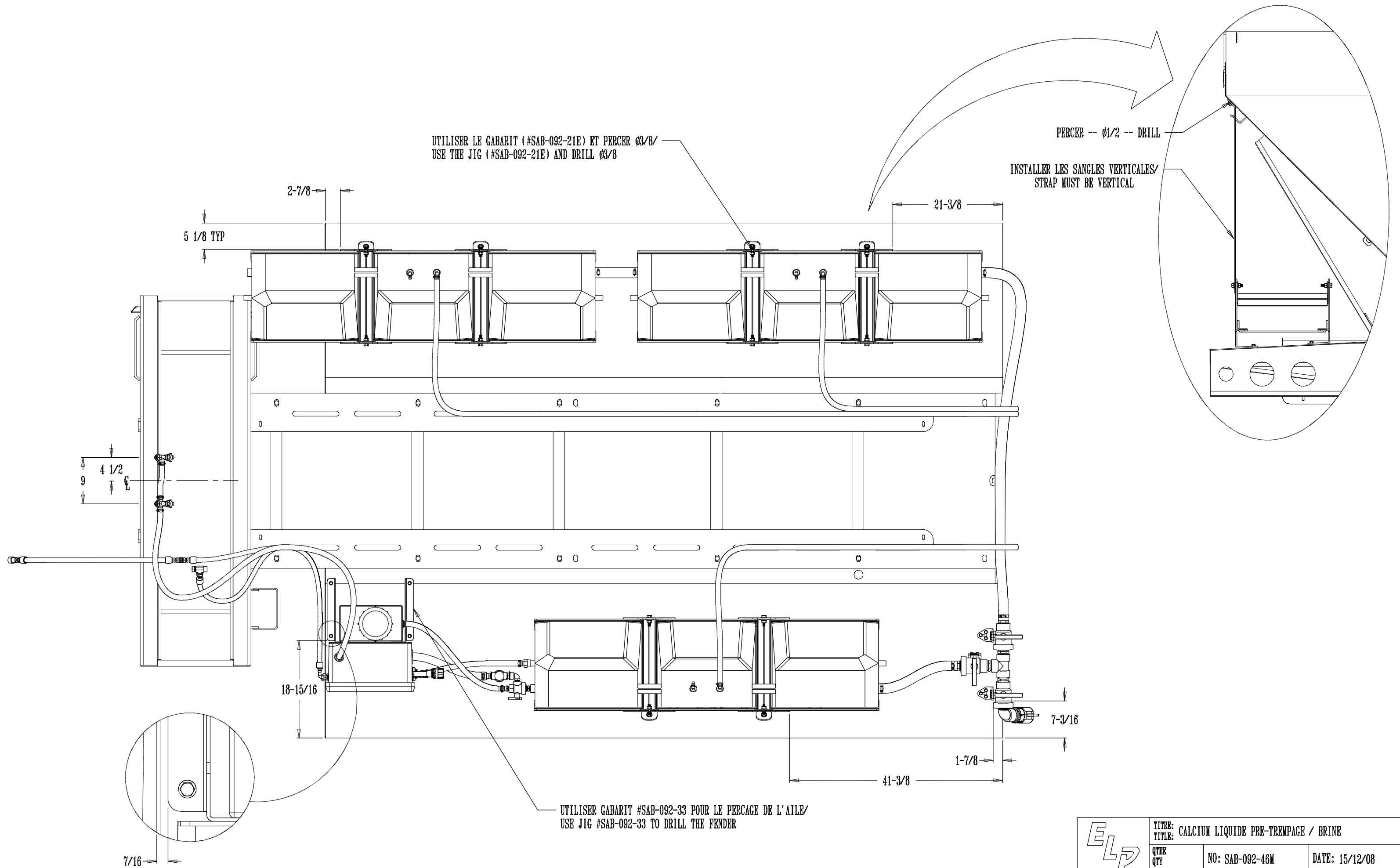
POSITION DES ELEMENTS / PARTS POSITIONNING
